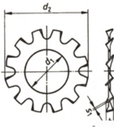
DIN 6797 A
