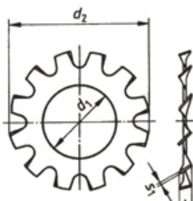
DIN 6797 A
