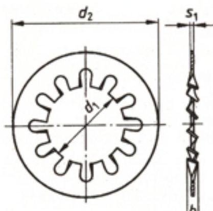
DIN 6797 J
