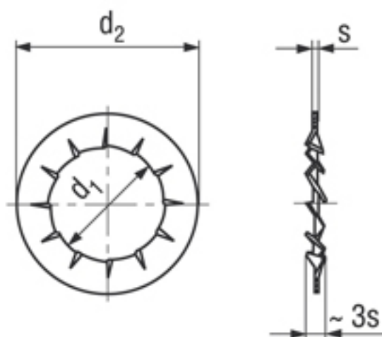
DIN 6798 J
