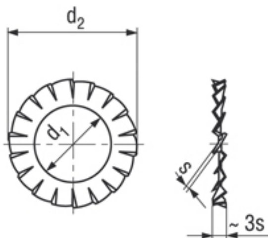
DIN 6798 A
