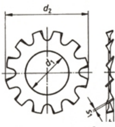
DIN 6797 A
