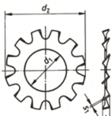
DIN 6797 A
